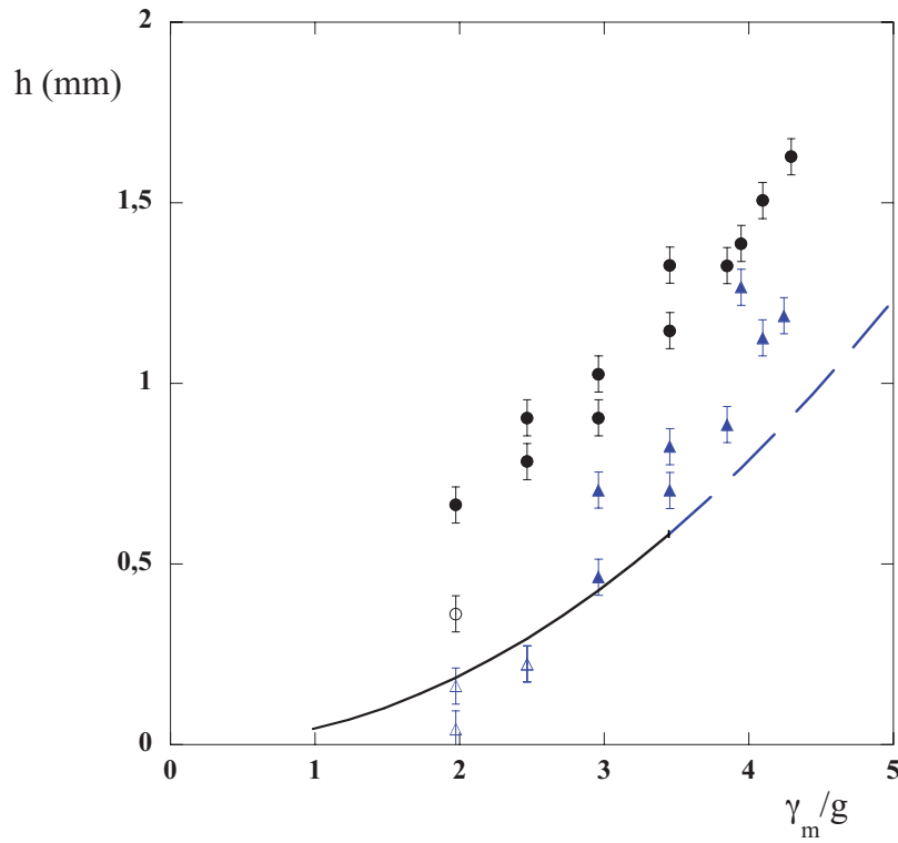
FIG. 3.6 – Les différents points correspondent à différents diamètres de gouttes : les ronds : D \approx 0.6 mm, les triangles : D \approx 1 mm. Points vides : la goutte effectue un rebond simple, points remplis : la goutte effectue un doublement de période. f_0 = 50 Hz, \mu_L = 50 \cdot 10^{-3} Pa.s. La courbe correspond à la hauteur théorique calculée pour f_0 = 50 Hz, avec en trait plein, le rebond simple et en pointillé le doublement de période.
