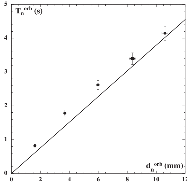
FIG. 5.10 – Période des orbites T_n^{\text{orb}} en fonction de la distance d_n^{\text{orb}} entre les deux gouttes identiques en rotation de la figure 5.8. La ligne correspond à la période qu'on observerait si les marcheurs maintenaient leur vitesse de marcheurs "libres" lorsqu'ils sont en orbite.
