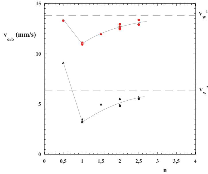
FIG. 6.20 – Vitesses de deux gouttes de taille différentes en fonction de la distance sur laquelle elles orbitent. En pointillé, la vitesse des gouttes en marcheur seul : v_W^1 = 6.35 mm/s et v_W^2 = 13.76 mm/s. En gris, les lignes servent de guide pour l'oeil. \mu_L = 20 \cdot 10^{-3} Pa.s, f_0 = 80 Hz, \gamma_m/g = 3.95 .
