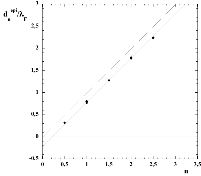
FIG. 6.19 – Pour une paire de deux gouttes différentes faisant des trajectoires épicycloïdales : d_n^{epi} / \lambda_F en fonction du paramètre d'ordre n .
